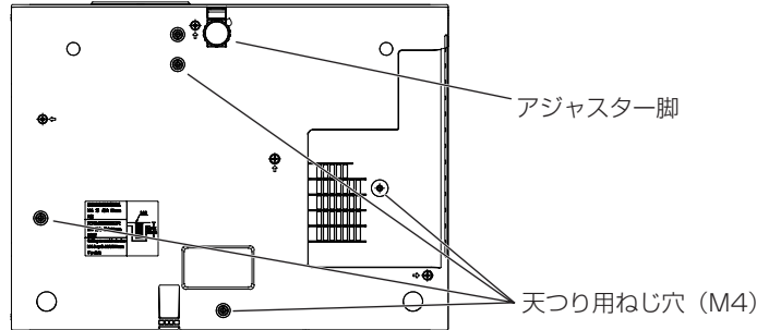
天つり用ねじ穴とアジャスター脚の位置
